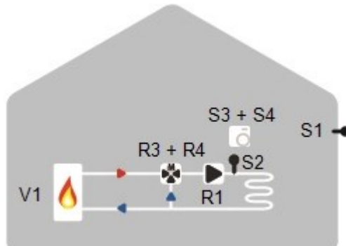
Gemischter Heizkreis mit Wärmeanforderung
